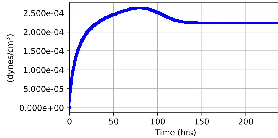
\Sigma |\vec{j} \cdot \vec{B}|
